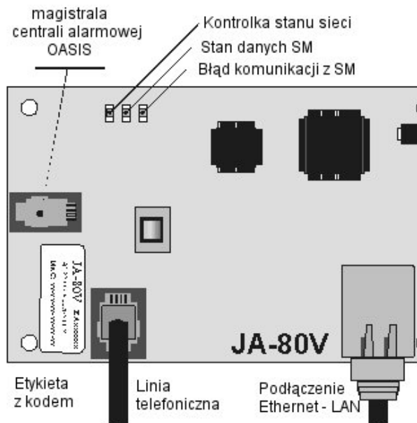
Rys. 1 Podłączenie dialera
