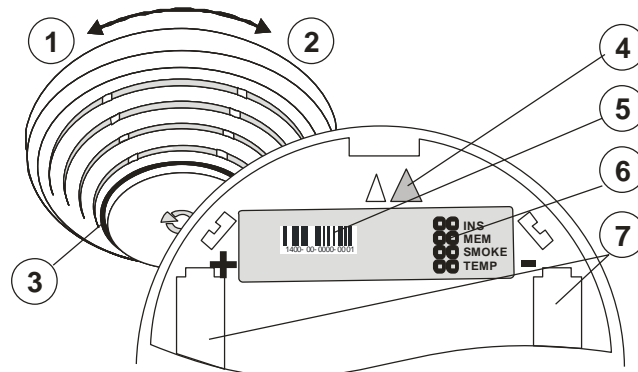
Rys. 1: 1 – otwieranie pokrywy czujnika; 2 – zamykanie pokrywy czujnika; 3 – sygnalizacja statusu optyki; 4 – strzałka wskazująca lokalizację czujnika; 5 – kod produkcji; 6 – zaciski konfiguracji; 7 – uchwyt baterii
