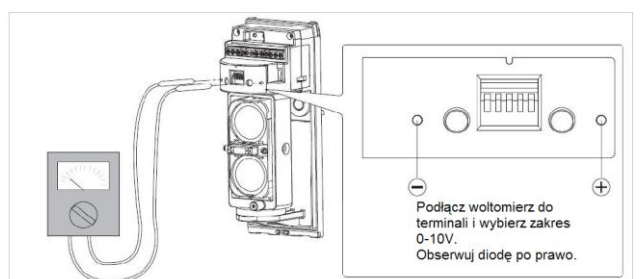
Rys. 6 Konfiguracja przy pomocy miernika uniwersalnego
